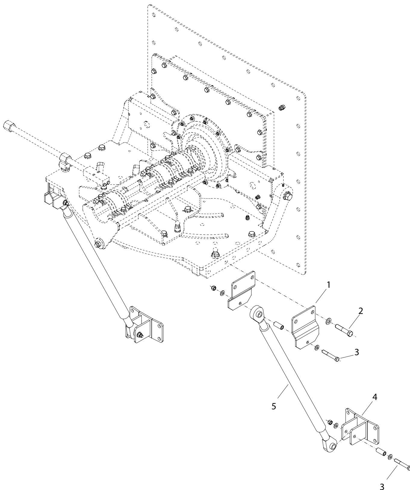
Abb. 7: Rührgigant FR SP mit Oberlenker unten Giantmix FR SP with upper link below
