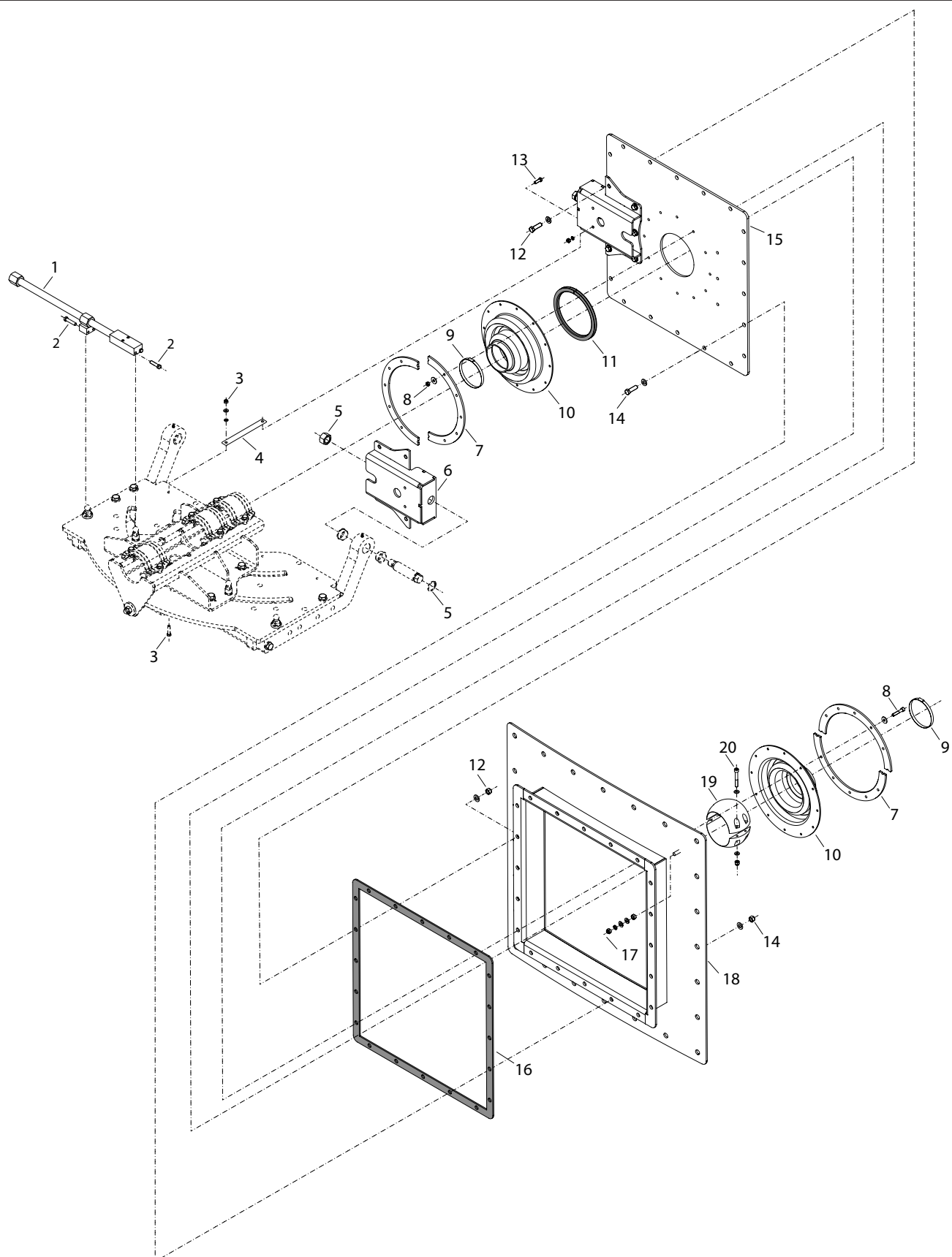
Abb. 5: Dichtplatte mit Schwenkeinrichtung Sealing plate with articulated frame
