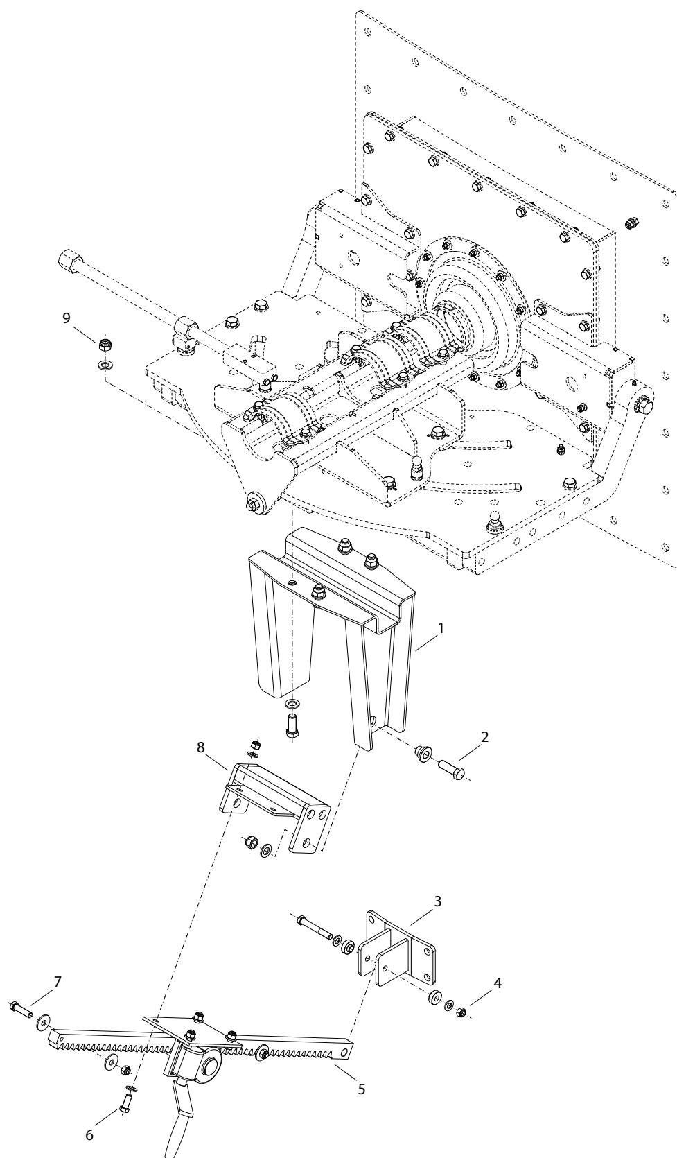
Abb. 9: Rührgigant FR SP mit Zahnstange unten Giantmix FR SP with pinion rack below
