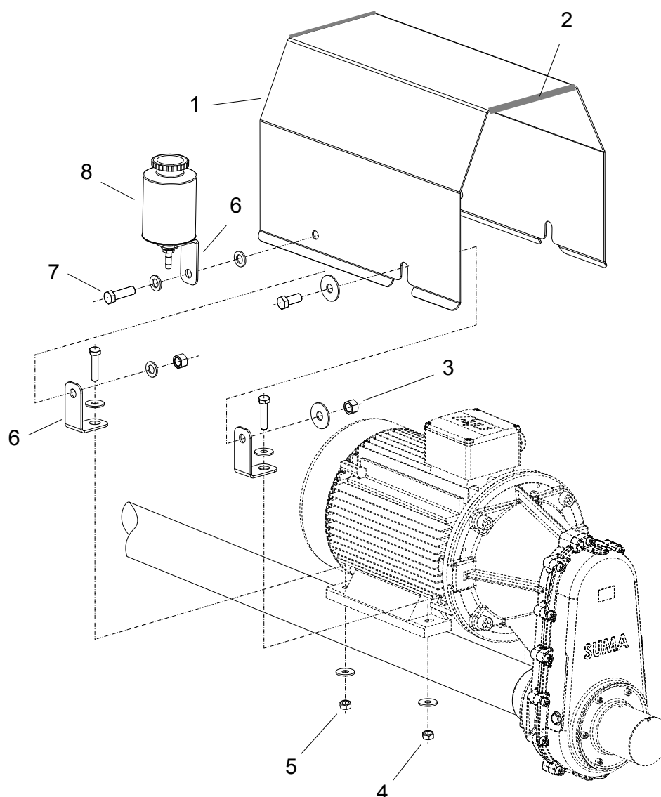
Abb. 13: Schutzhaube für Elektromotor (Option) Protective hood for electric motor (option)
