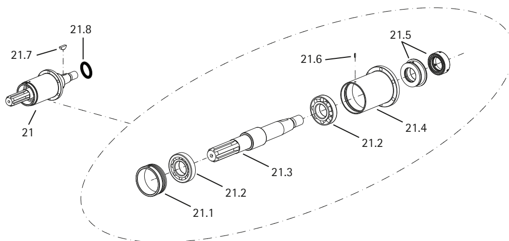
Abb. 3: Lagergehäuse komplett, mit Gleitringdichtung (GLRD) Bearing housing assy., with axial face seal (GLRD)
