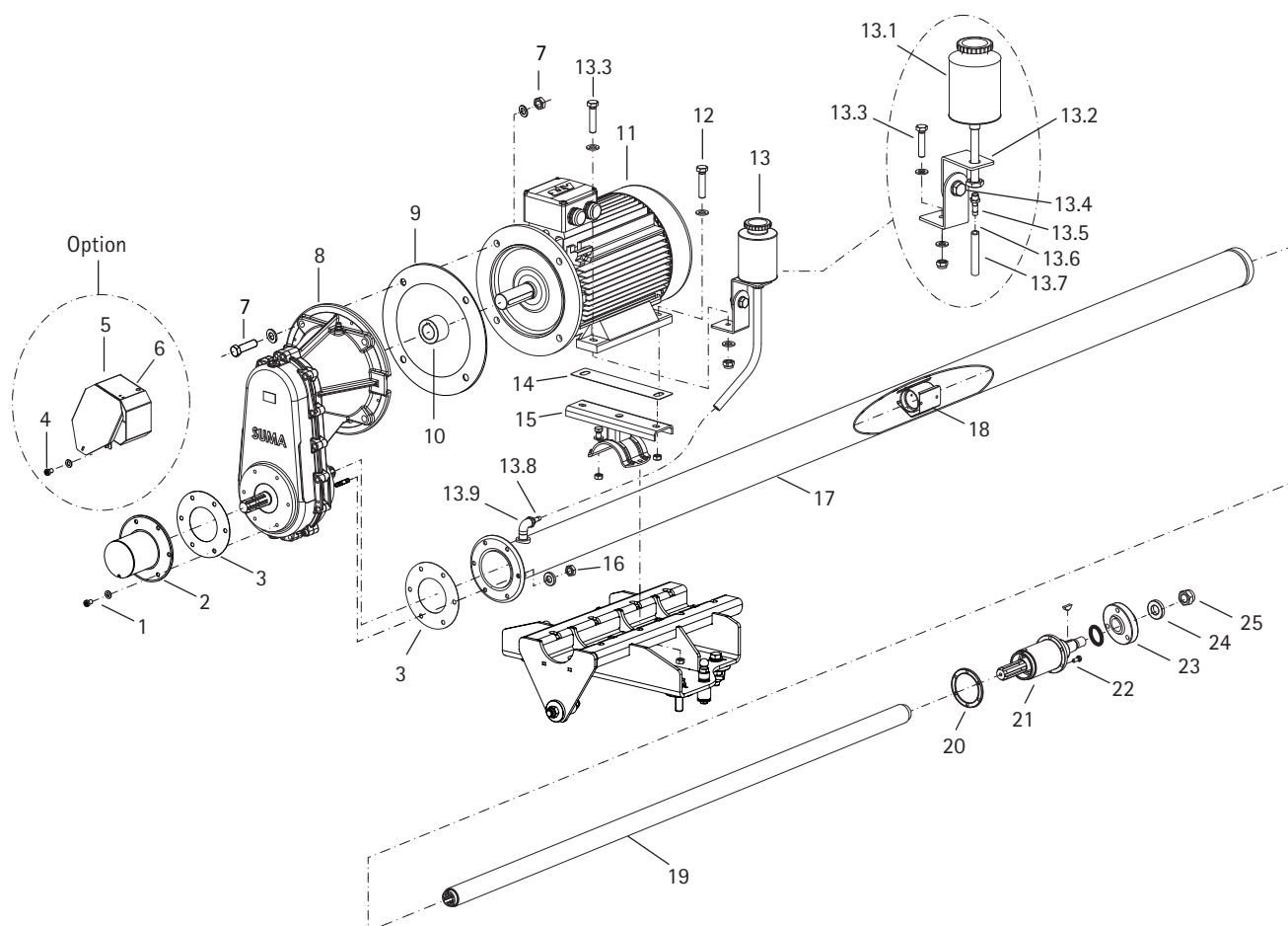
Abb. 2: Rührwerkrohr komplett mit Kombigetriebe FR SP Agitator shaft tube assembly with combined transmission FR SP
