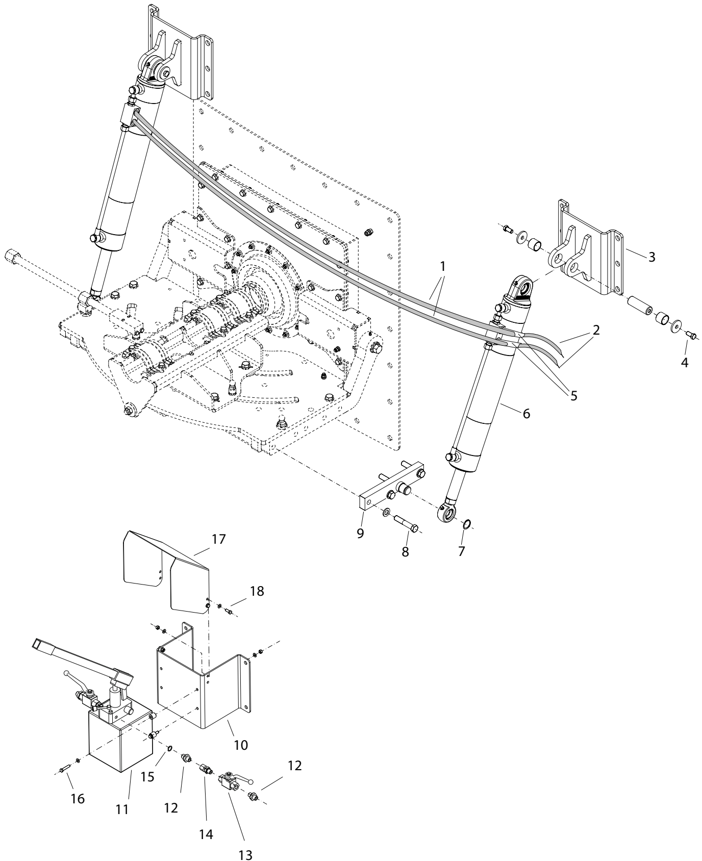
Abb. 12: Rührgigant FR SP mit Hydraulikzylinder oben Giantmix FR SP with hydraulic cylinder above
