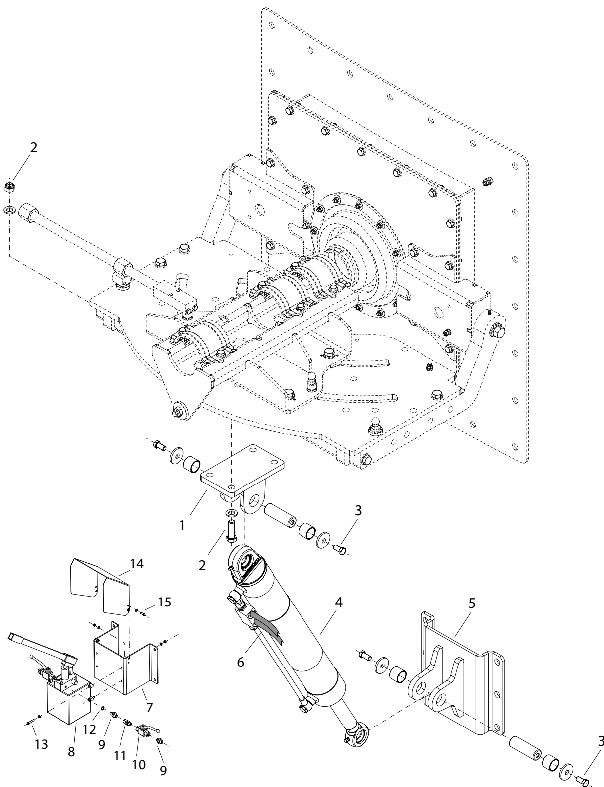
Abb. 11: Rührgigant FR SP mit Hydraulikzylinder unten Giantmix FR SP with hydraulic cylinder below
