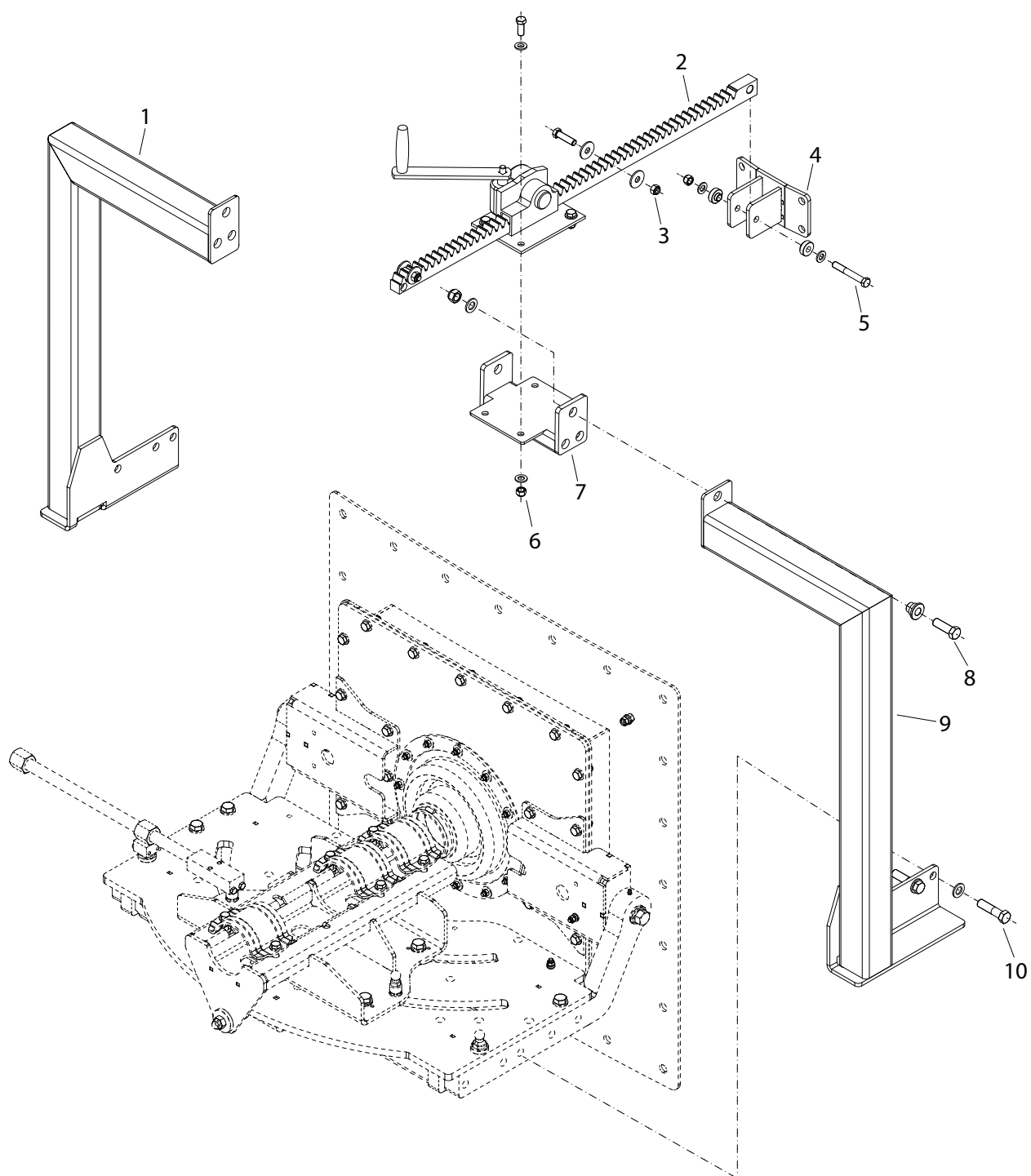
Abb. 10: Rührgigant FR SP mit Zahnstange oben Giantmix FR SP with pinion rack above
