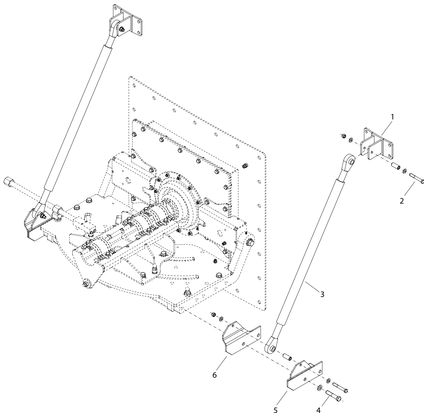
Abb. 8: Rührgigant FR SP mit Oberlenker oben Giantmix FR SP with upper link above
