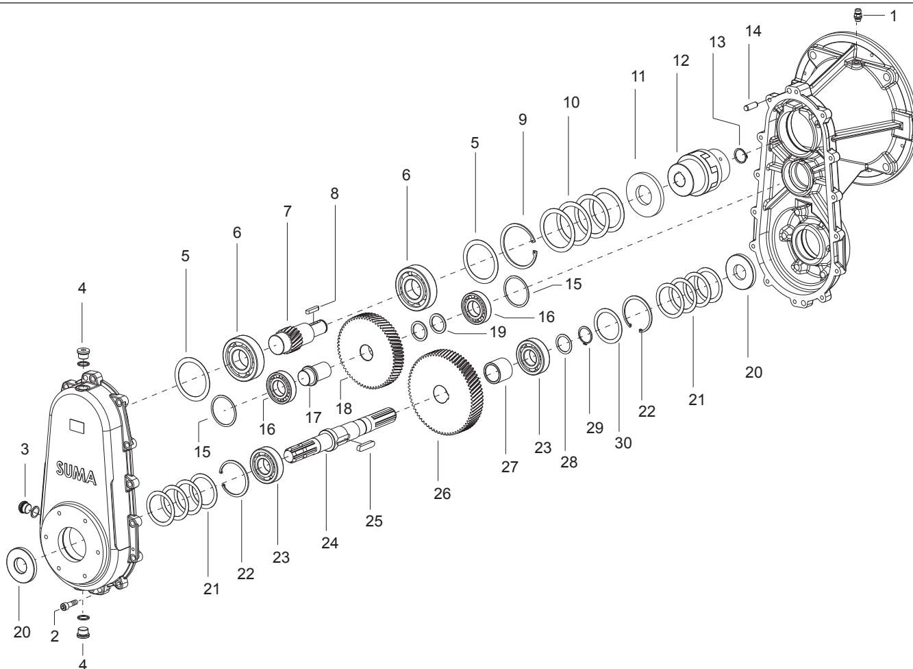
Abb. 4: Stirnradgetriebe Rührigigant FR: i=3,69 / i=5,31 (LL) Spur gearing Giantmix FR: i=3,69 / i=5,31 (LL)
